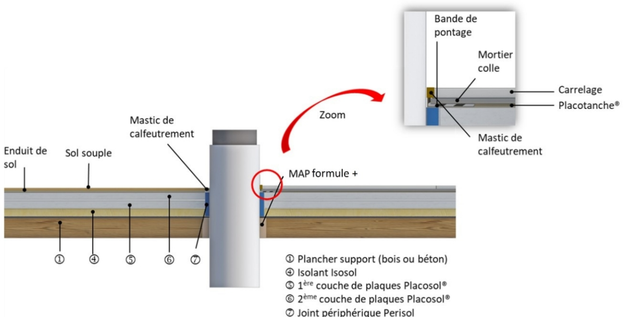
Figure 7 - Dispositions de mise en œuvre de la chape sèche au droit des pénétrations
