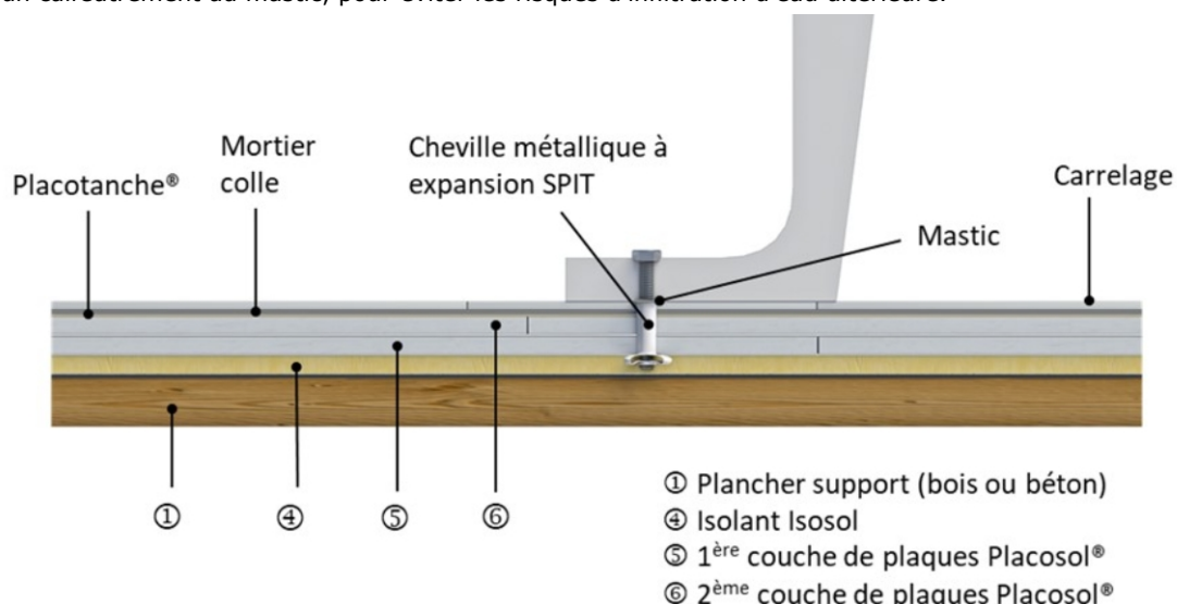
Figure 8 - Dispositions de mise en œuvre de la chape sèche dans le cas d'un appareil sanitaire
