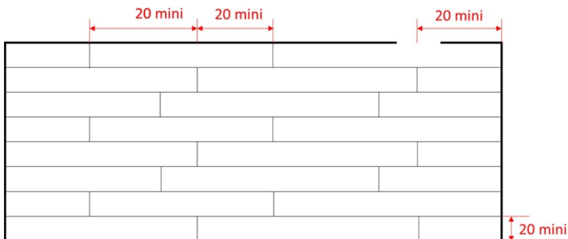
Figure 3 - Illustration pose 1 er lit de plaques Placosol® (cotes en cm)
