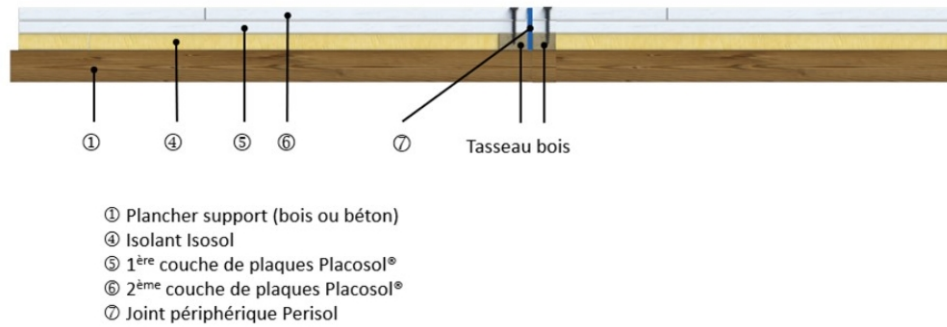
Figure 5d - Illustration des dispositions de mise en œuvre de la chape sèche en cas de joints de fractionnement (a) et (D), et de dilatation (b) et (c)
