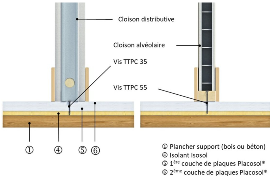
Figure 2 - Illustration des dispositions de mise en œuvre de cloison distributive et alvéolaire sur chape sèche
