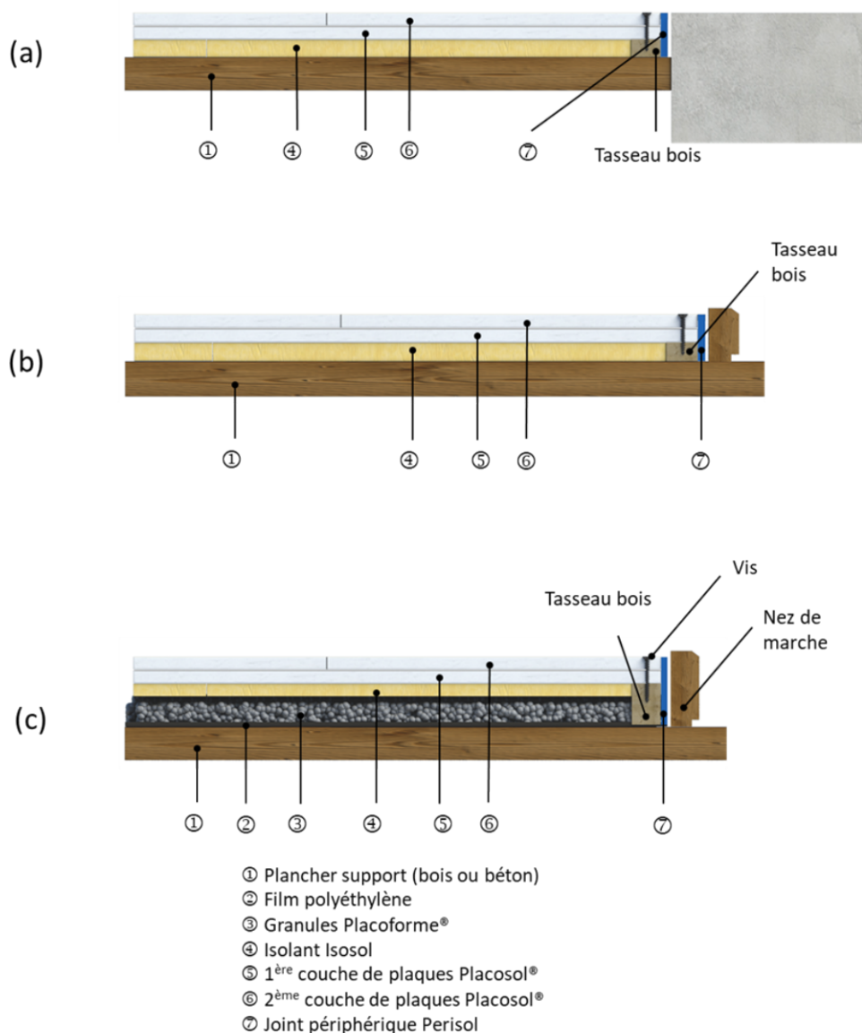
Figures 5a, 5b, 5c - Illustration des dispositions de mise en œuvre de la chape sèche en cas de joints de fractionnement changement de support (a) et (D), et de dilatation (b) et (c)
