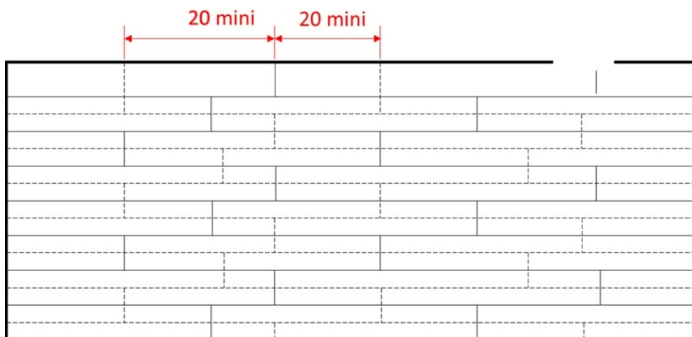
Figure 4 - Illustration 2 ème lit de plaques Placosol® (cotes en cm)
