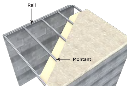
Plafonds autoportants sur rails et montants Stil®
