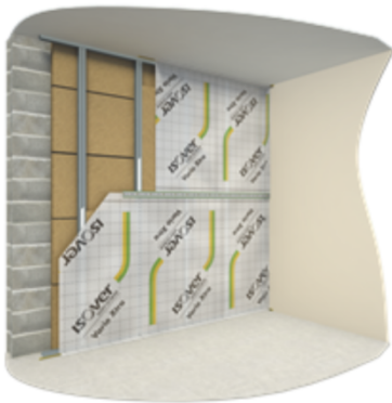
Figure 4-3: Mise en place de la membrane pare-vapeur Vario® Xtra sur l'ossature métallique à l'aide de double face
