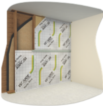
Figure 5-2 bis : Variante de pose de la membrane Vario® Xtra via agrafage sur montants bois et une seule couche d'isolant
