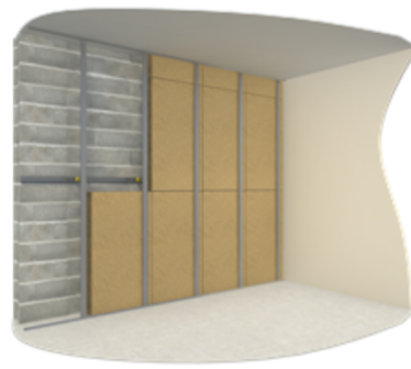
Figure 3-2 : Insertion des panneaux ISONAT FLEX derrière l'ossature métallique
