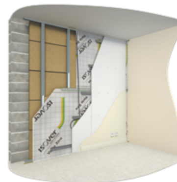
Figure 4-4 : Mise en place des profilés métalliques Stilmob et des gaines électriques (Hors ERP)
