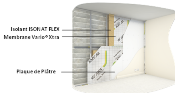
Figure 3-5 : Pose des plaques de plâtre en ERP
