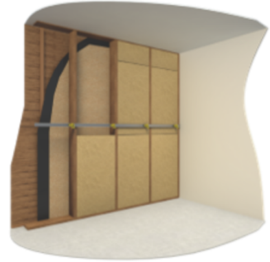
Figure 5-2 : Installation de la fourrure intermédiaire et des appuis Optima 2 clipsés sur fourrure
