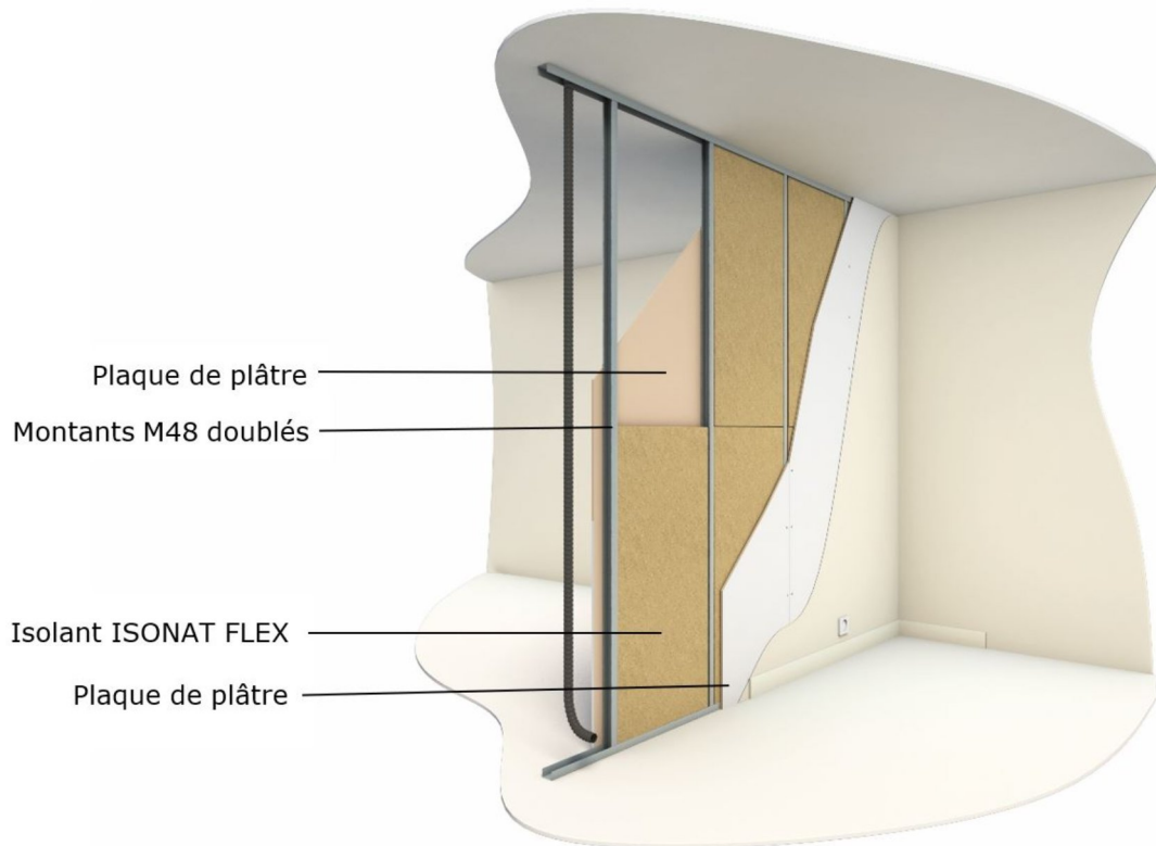
Figure 1 : Réalisation d'une cloison sur ossature métallique avec montants M48 simples
