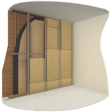
Figure 5-3 : Pose des fourrures métalliques verticales et de la seconde couche d'isolation entre fourrures.
