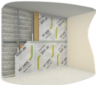
Figure 3-3 : Mise en place de la membrane pare-vapeur Vario® Xtra sur l'ossature métallique à l'aide de double face
