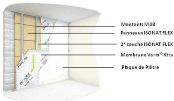
Figure 4-5 : Pose des plaques de plâtre en ERP
