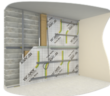
Figure 3-4 : Mise en place des profilés métalliques Stilmob et des gaines électriques (Hors ERP)
