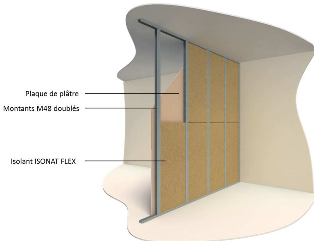
Figure 2 : Réalisation d'une cloison sur ossature métallique avec montants M48 doublés
