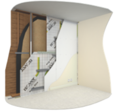
Figure 5-4 : Pose de la membrane Vario® Xtra à l'aide de double face puis installation des Stilmob puis celle de la plaque de plâtre
