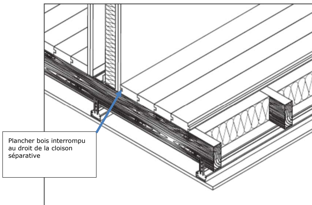
Figure 3 - Raccordement sur plancher bois avec interruption du platelage pour atténuation des transmissions latérales.
