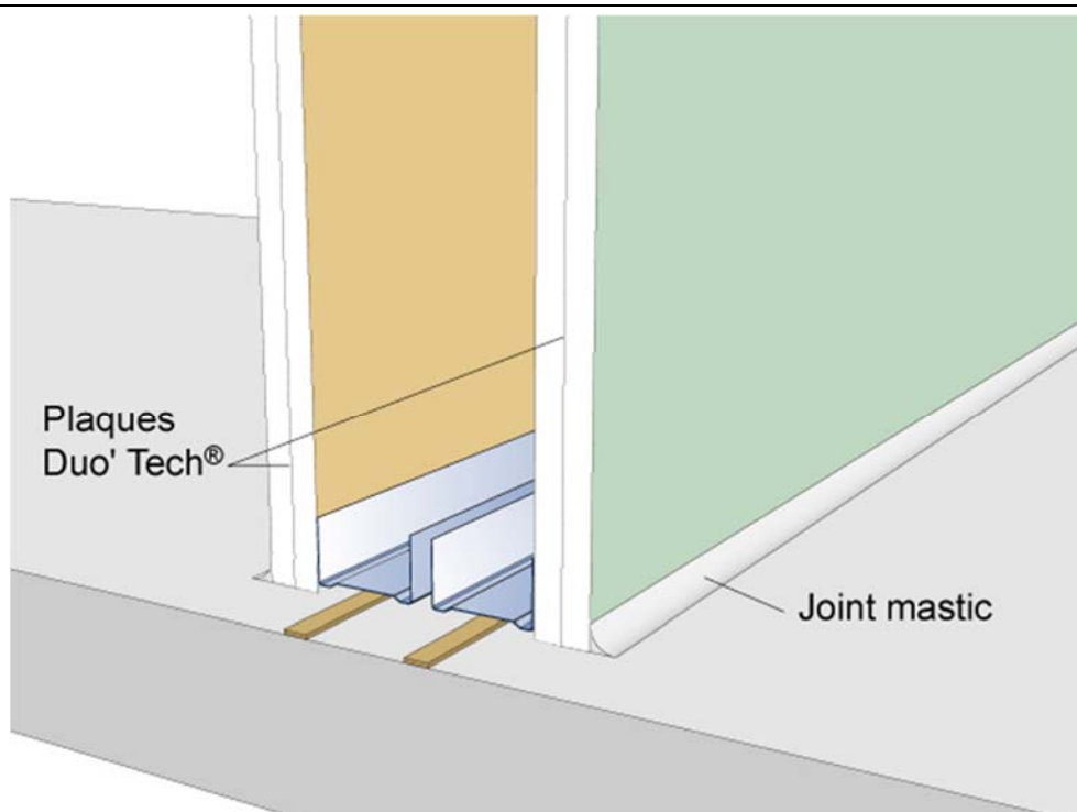
Figure 5 - Dispositions en pied de cloison en locaux EB+ Privatifs
