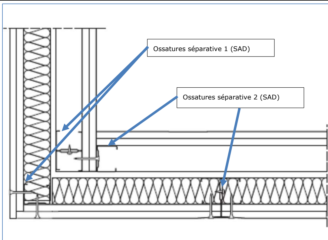
Figure 6 - Jonctions en L avec une autre séparative (coupe horizontale)
