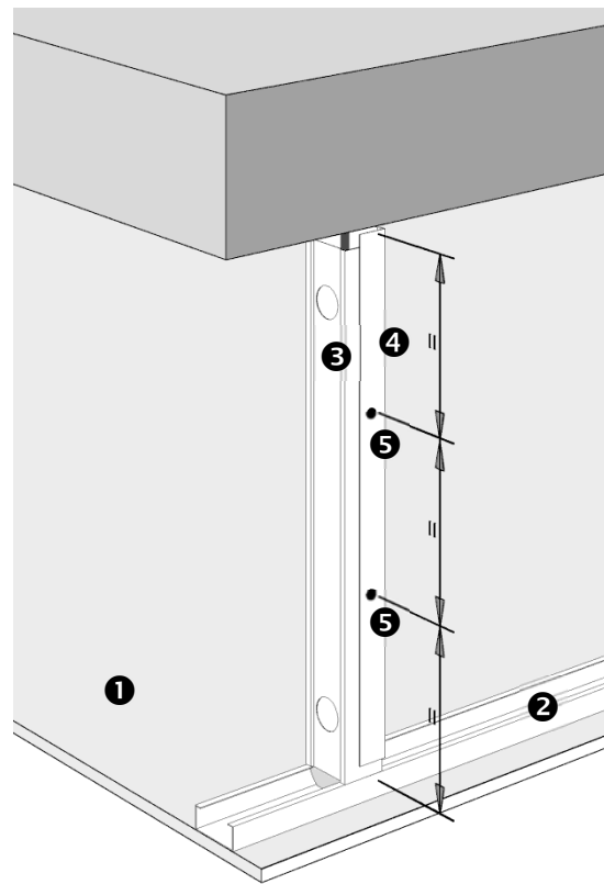
Figure 3 – Positionnement des vis TRPF 13 sur bouton de longueur inférieure ou égale à 1m
