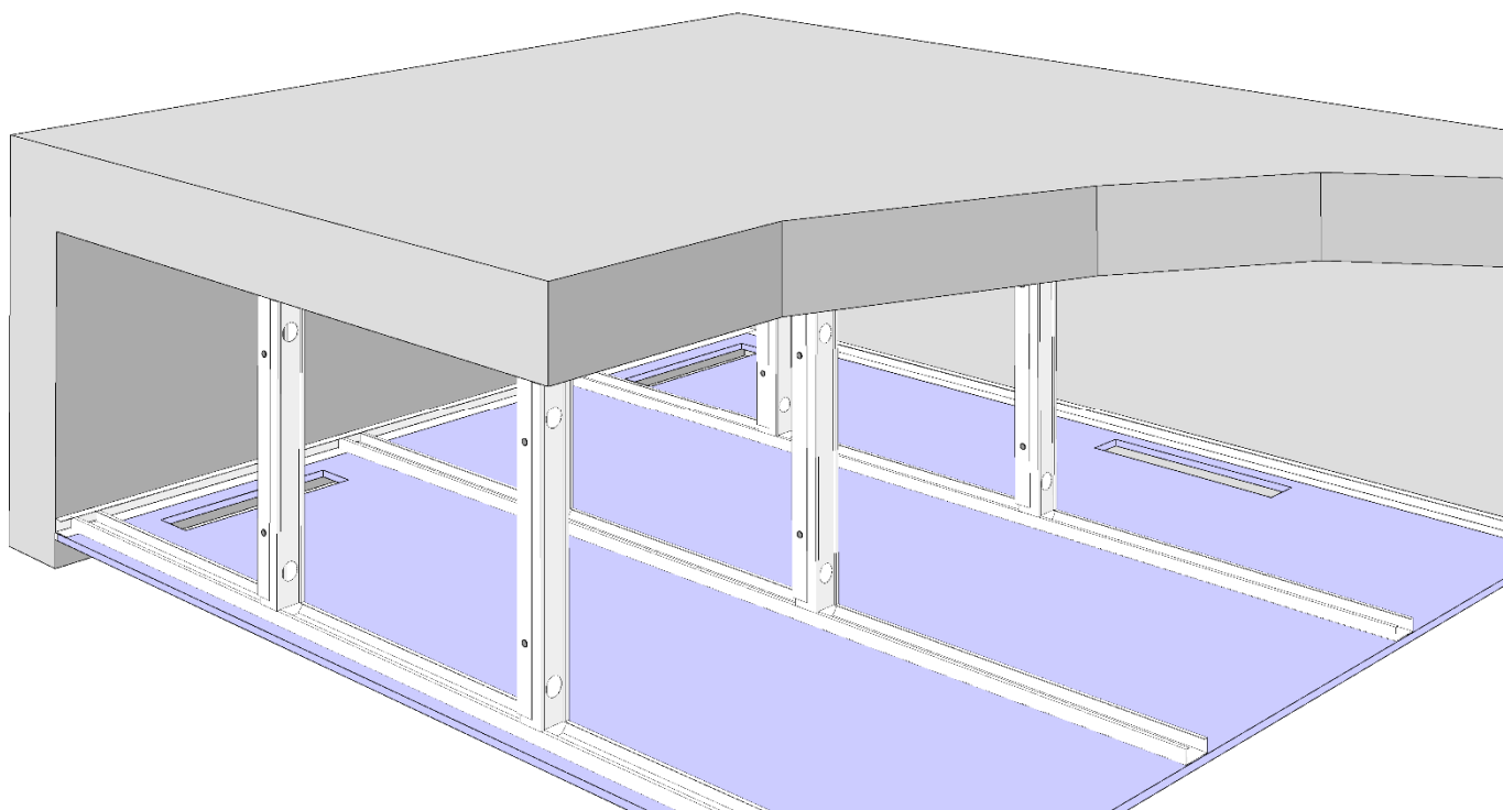
Figure 5 – Traitement de la périphérie du plafond et orifices de ventilation du plénum
