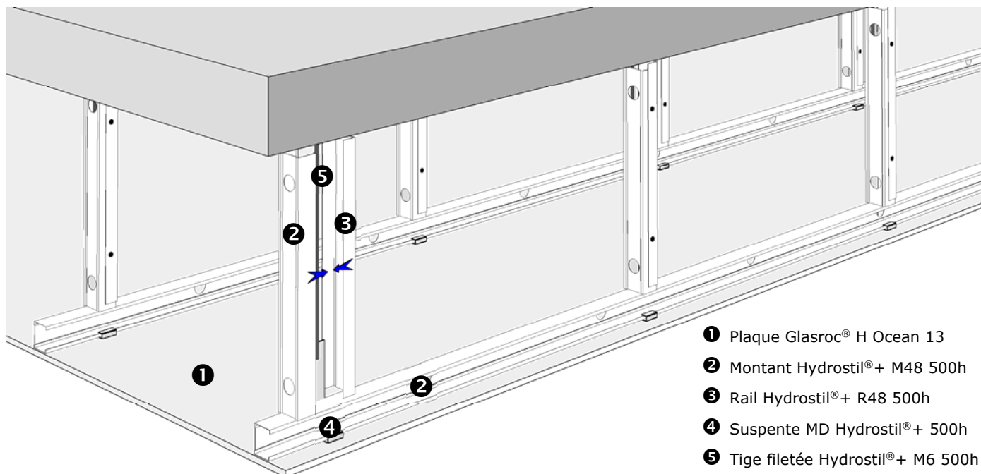
Figure 2 – Plafond Glasroc® H Ocean sur montants simples avec butonnage (plénum compris entre 30 cm et 1,5 m)
