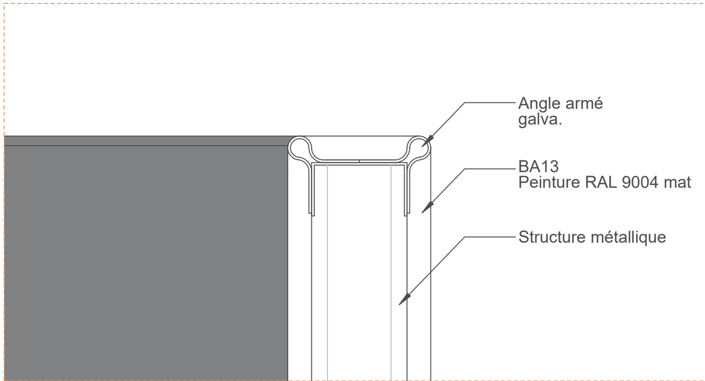
DET 2. TETE GARDE-CORPS 1/5
