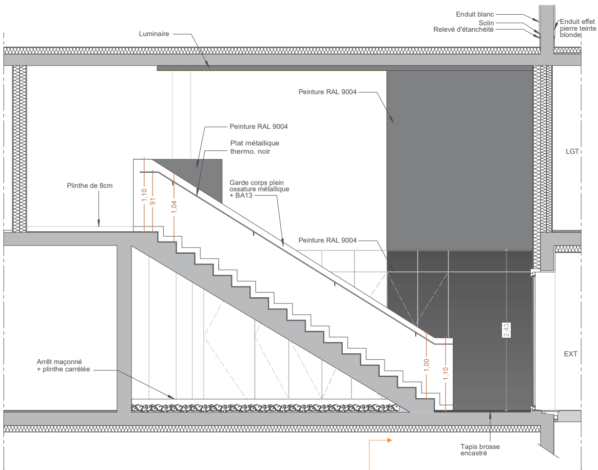
COUPE BB 1/50
