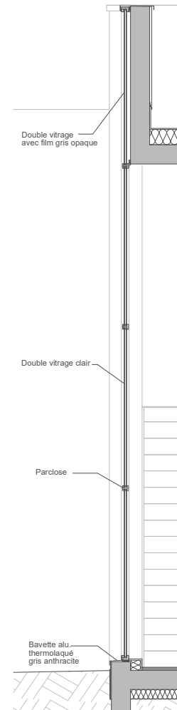
COUPE DD 1/50
